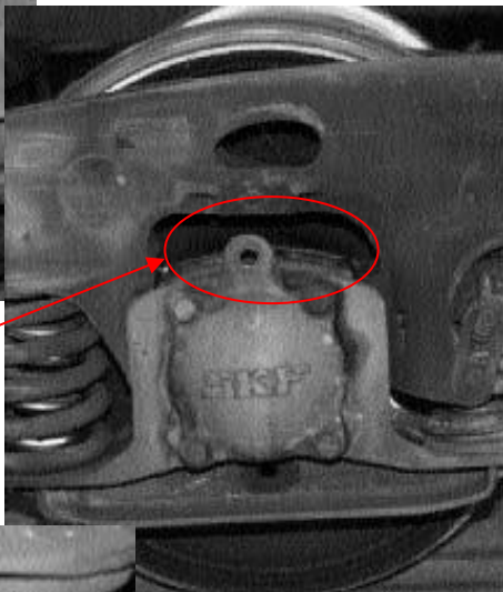
Fig. 6 Sécurité de relevage perdue
