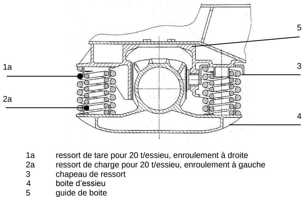
Figure 1 – Bogie avec ressorts pour une charge de 20 t/essieu
