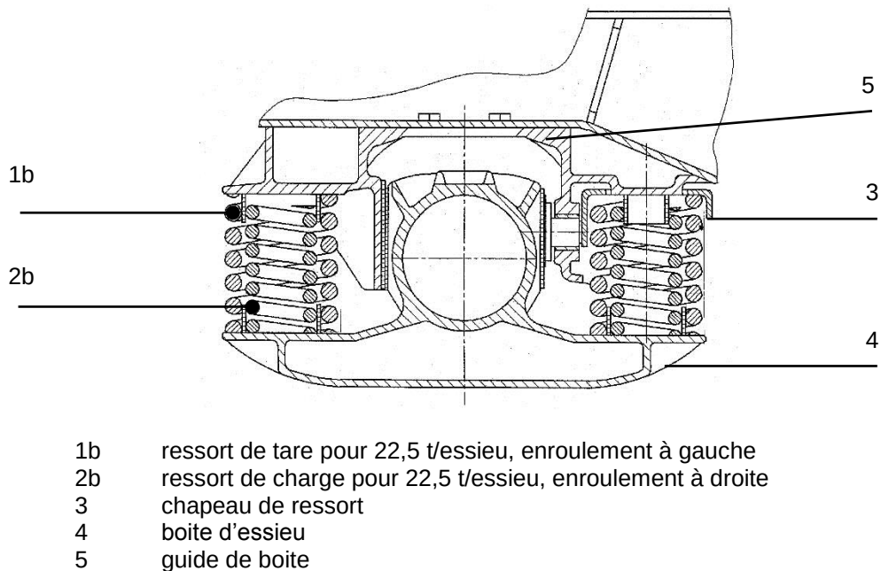
Figure 2 – Bogie avec ressorts pour une charge de 22,5 t/essieu
