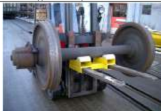
Photo 7 : Support d'essieu pour chariot à fourches (chargé)
