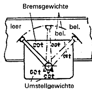
Bild 2 Abbremsung des Eigengewichts und mehrere (zum Beispiel zwei) Lastabbremsstellungen
